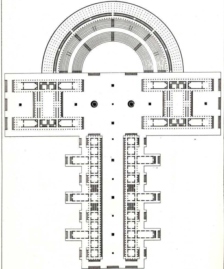
ENSEMBLE FORME PAR LA COMBINAISON DE PLUSIEURS EDIFICES.
